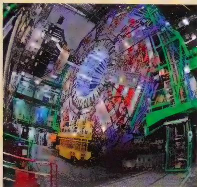
El detector ATLAS del acelerador del CERN está diseñado para estudiar partículas subatómicas, incluidas las predichas por la teoría de grupos.
